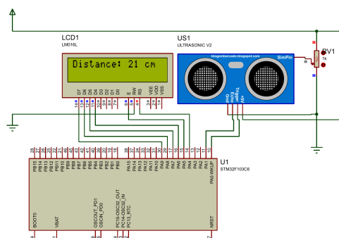
(ت) محاسبه فاصله ۲۱ سانتی‌متر
