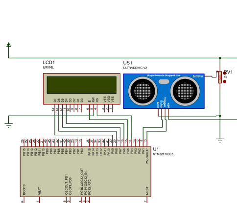
(ب) شماتیک مدار سنسور آلتراسونیک در پروتئوس
