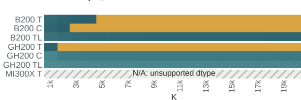
matmul · fp8_e4m3fn
