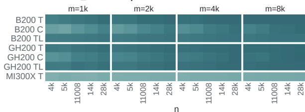
streamk_matmul · fp16
