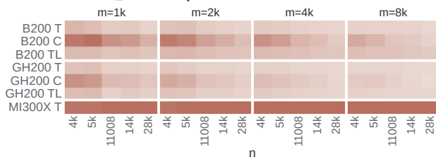
matmul · fp16
