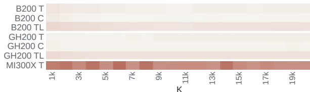
matmul · fp8_e4m3fn
