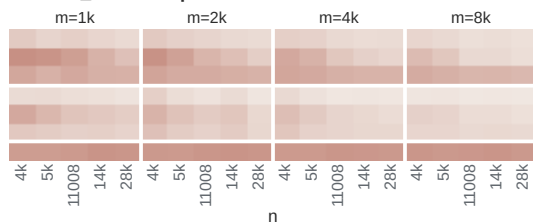
matmul · fp32
