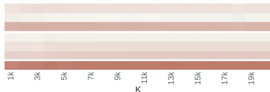
matmul · fp32
