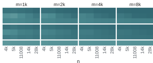
matmul · fp32
