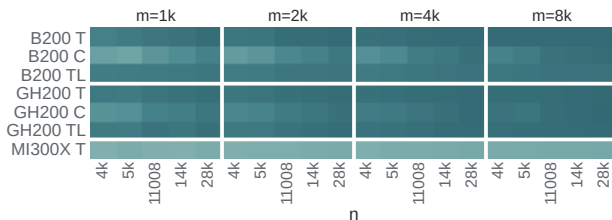
matmul · fp16
