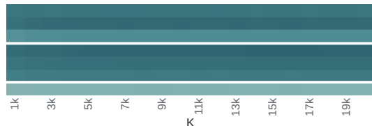
matmul · fp32
