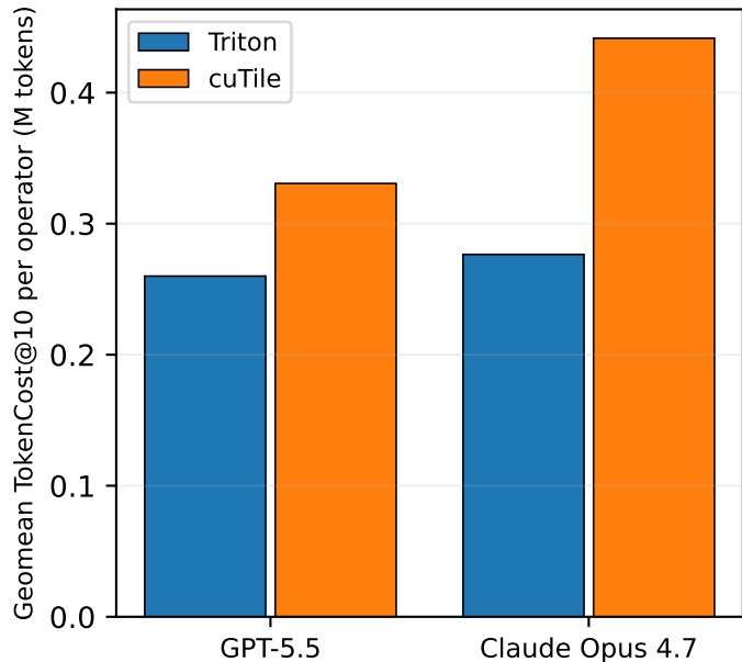
TokenCost@10
