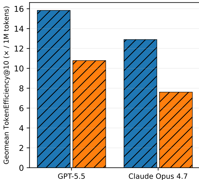
TokenEfficiency@10
