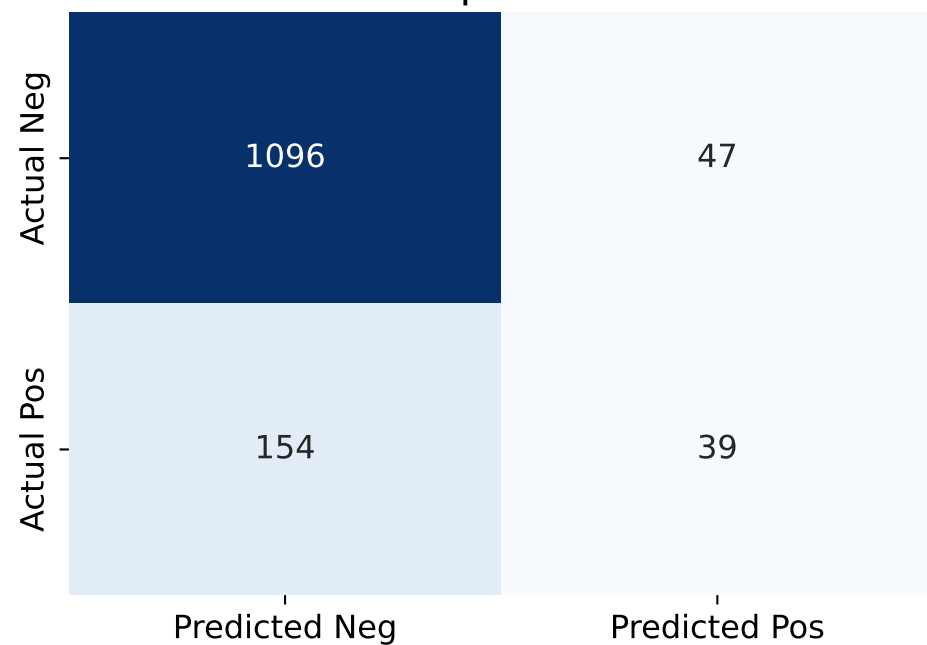
PPO-topk-mil-soft
