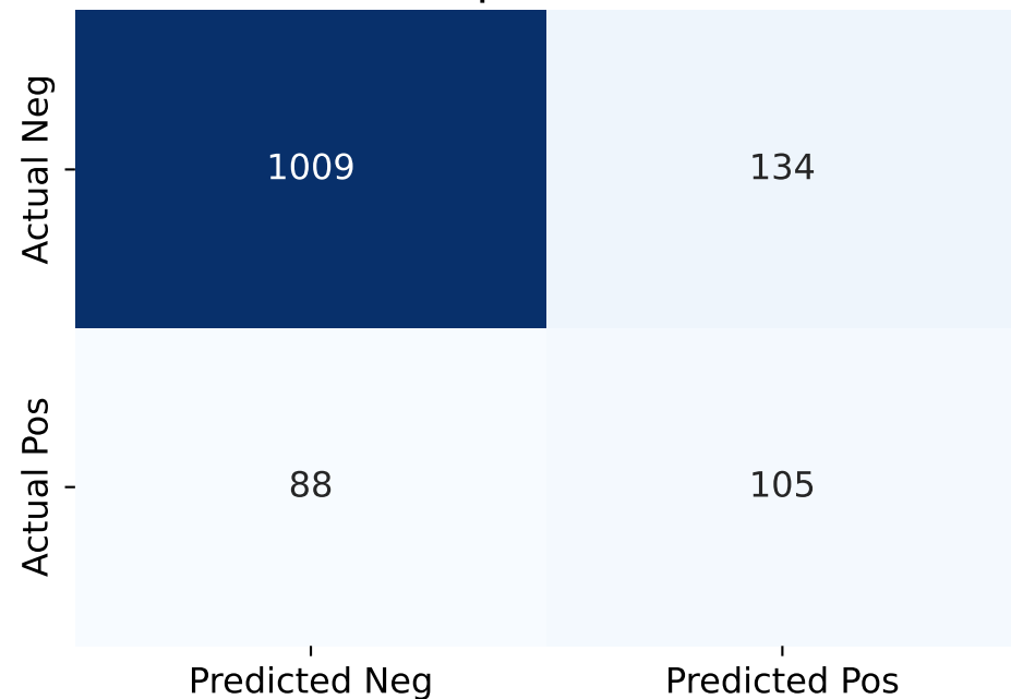
PPO-topk-mil-soft
