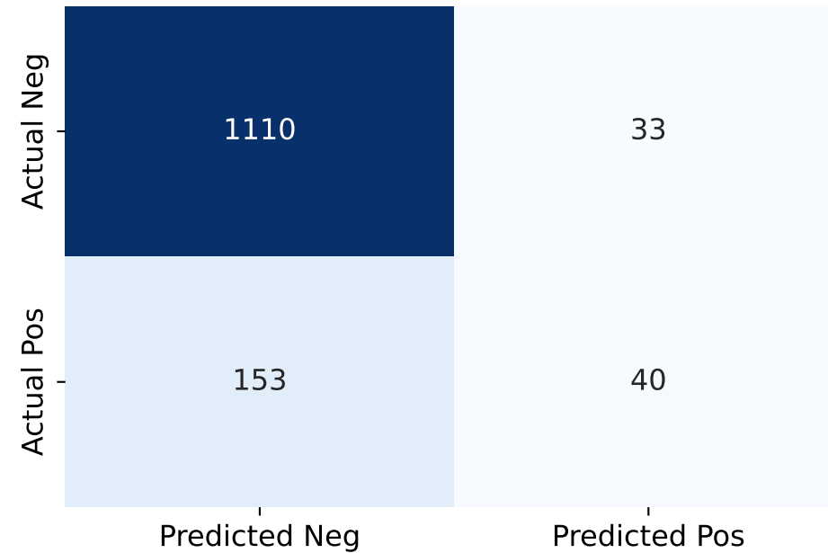
ProstNFound+v2
