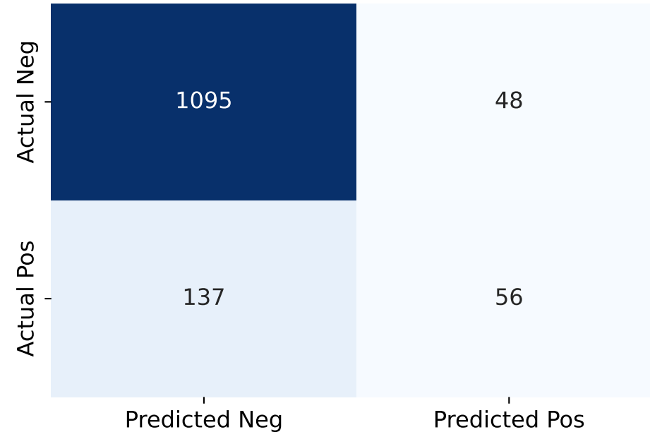
ProstNFound+v2
