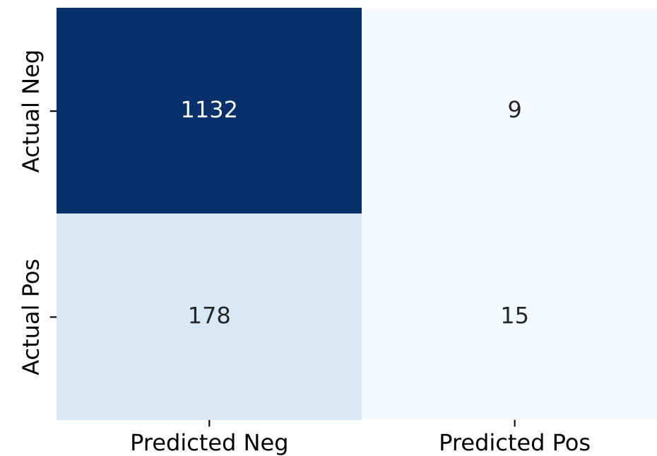
ProstNFound+
