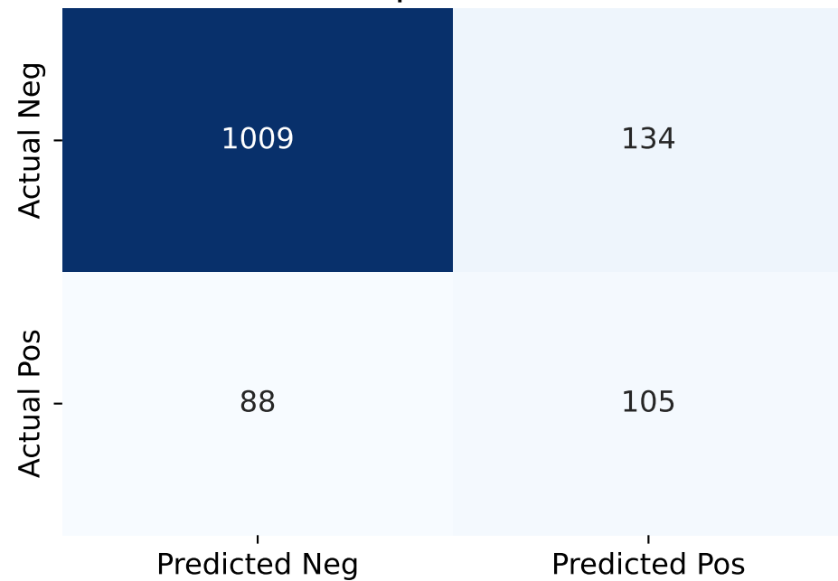
PPO+8
