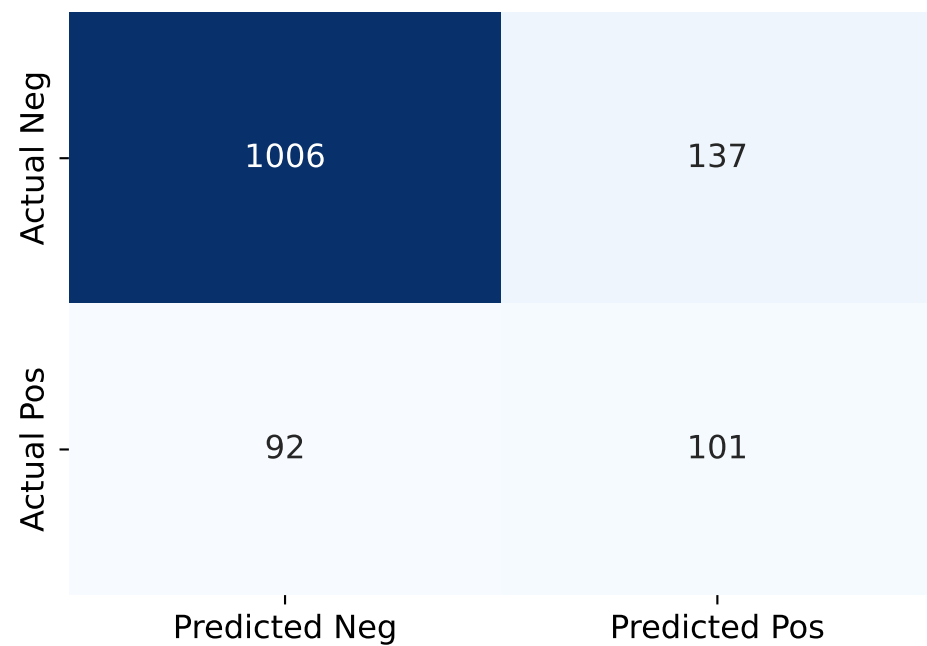
PPO+8
