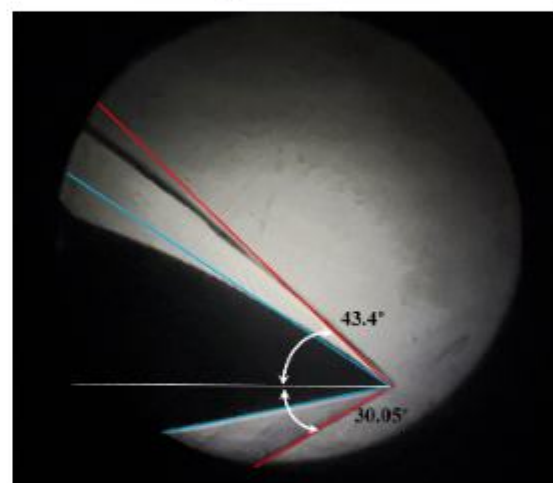
(d) 10° AoA
