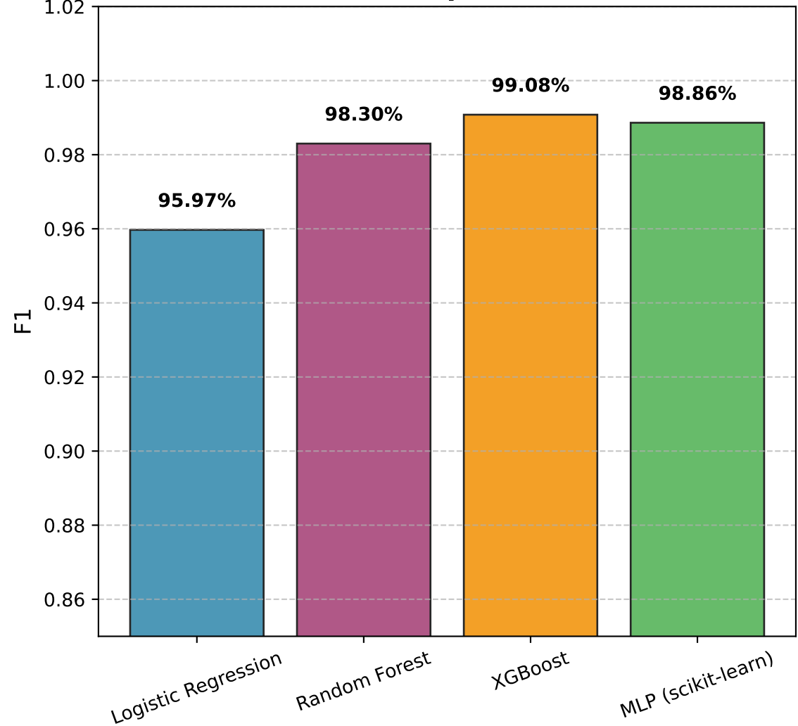
F1 Comparison
