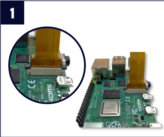
Raspberry Pi 4 ↔ FFC 케이블 연결 (15pin ↔ CAMERA 포트)
