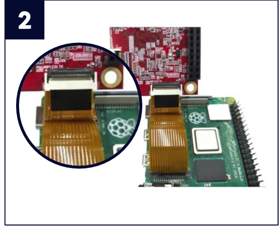
Raspberry Pi 4 연결된 FFC 케이블과 Tachy-Shield 연결(22pin ↔ J5 MIPI CSI TX)
