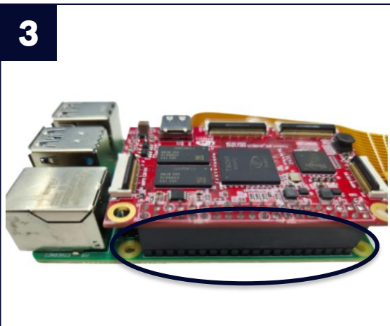
Raspberry Pi 4와 Tachy-Shield의 핀 헤더 결합
