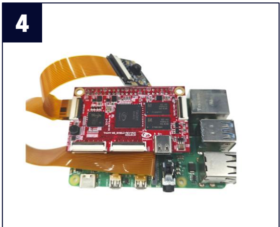
① MX219와 FFC 케이블 연결 (15pin ↔ J1) ② IMX219에 연결된 FFC 케이블과 Tachy-Shield간 연결(22pin ↔ J8 MIPI1 CSI RX)
