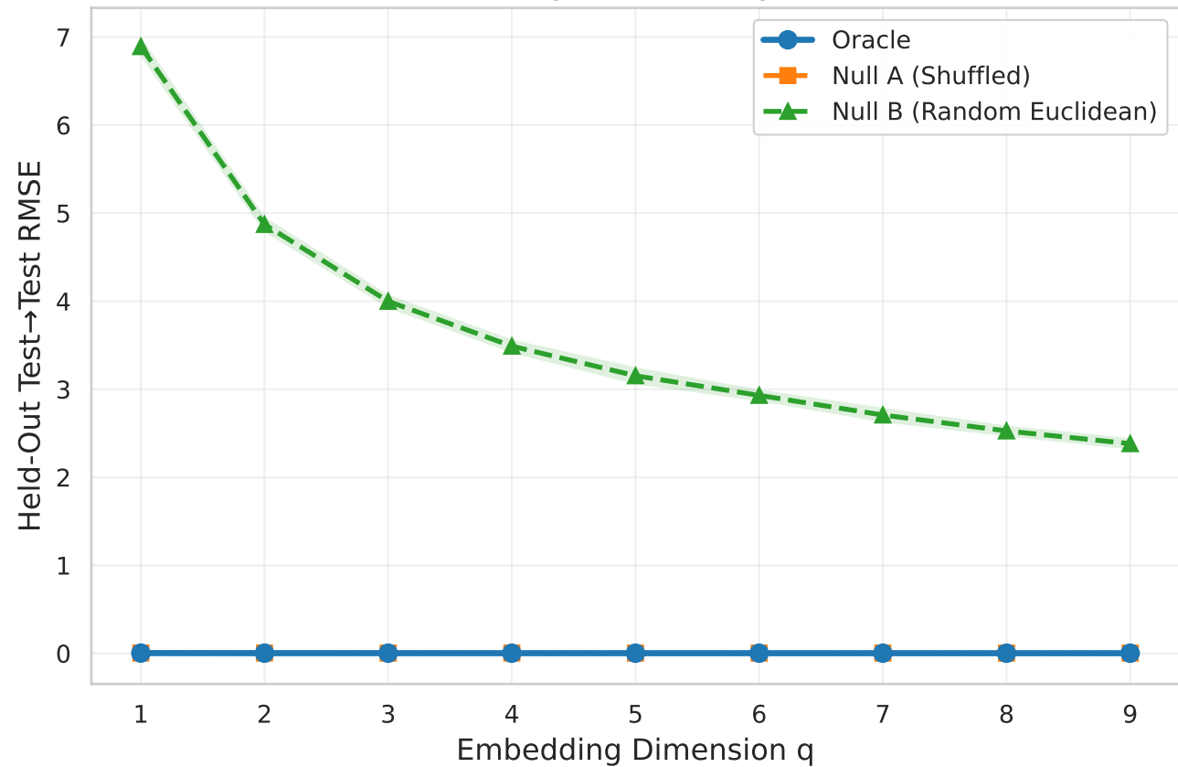
Embedding Error — Layer: last
