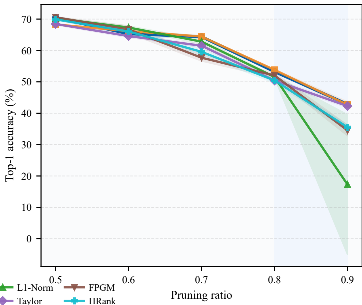
VGG-16 / CIFAR-100
