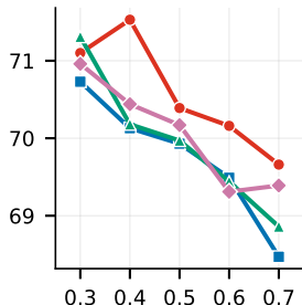
(j) ResNet-56
