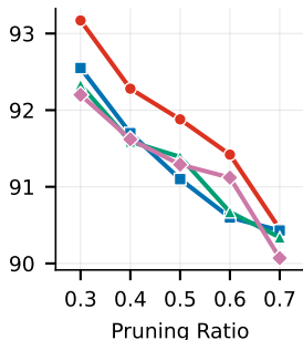
(j) ResNet-56
