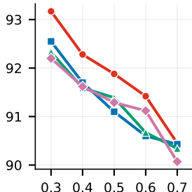
(f) ResNet-56
