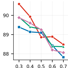
(h) VGG-16
