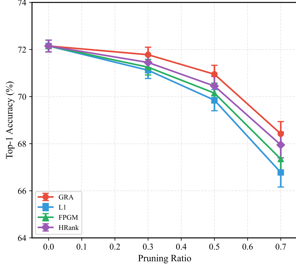
(d) ResNet-56/CIFAR-100: Accuracy vs Ratio
