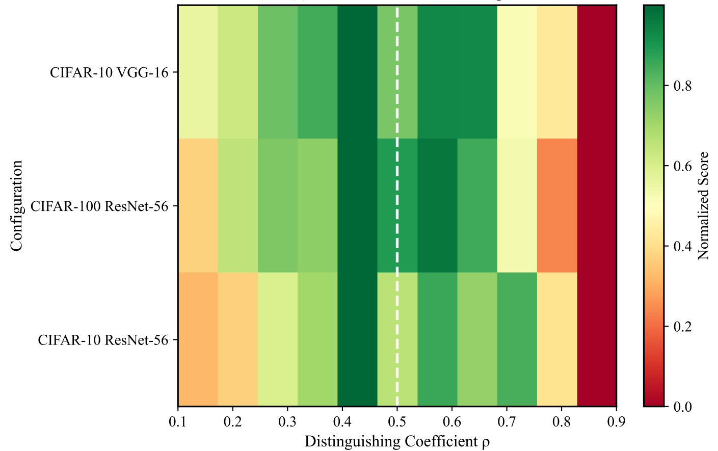
(d) Normalized Score Heatmap
