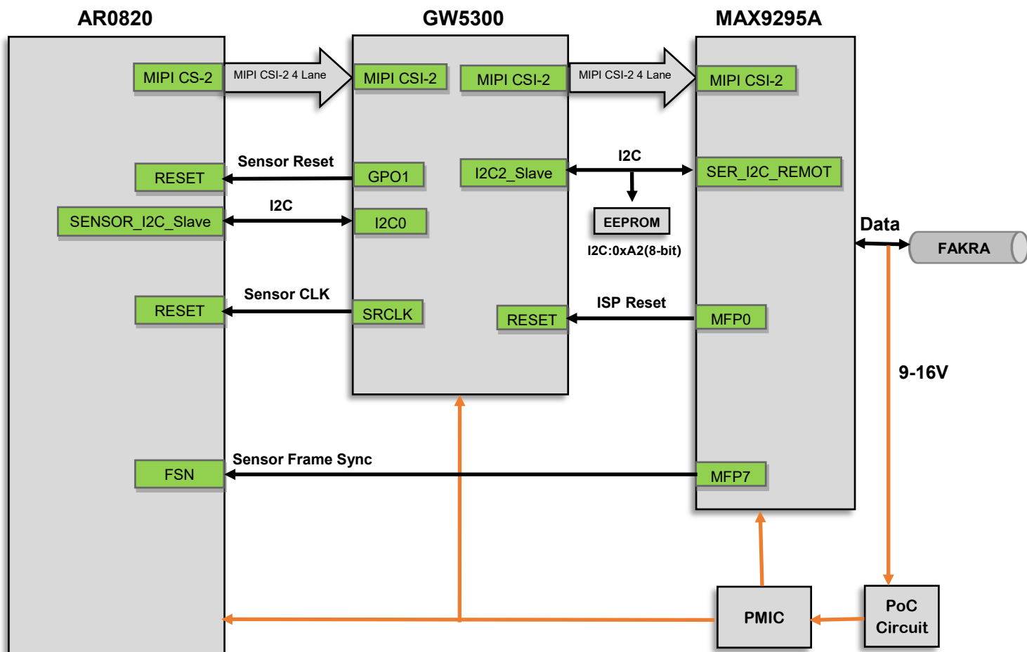
系统框图
