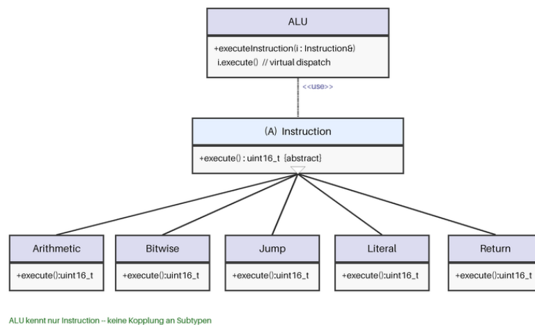
Abbildung 7.4: UML nach dem Refactoring: ALU kennt nur die abstrakte Schnittstelle Instruction ; konkreter Typ ist zur Kompilierzeit irrelevant.
