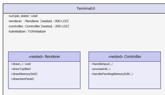
Abbildung 7.1: UML vor dem Refactoring: Renderer und Controller als Nested-Classes innerhalb von TerminalUI .
