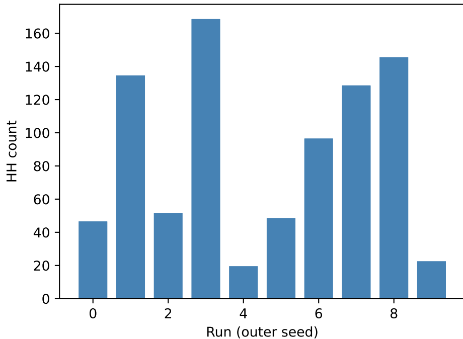
HH count per run (COMPAS)
