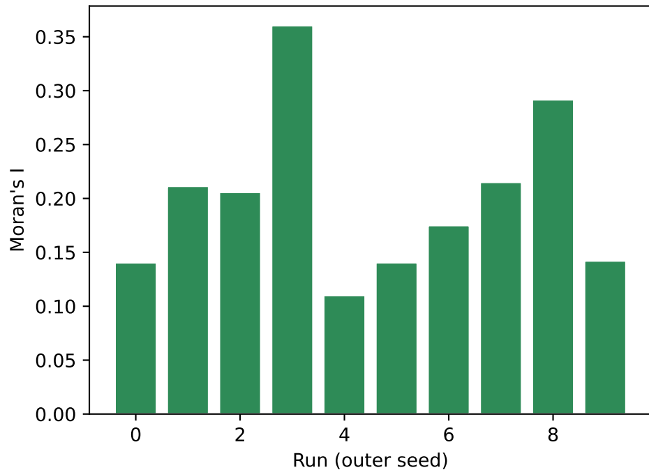
Moran's I per run (COMPAS)
