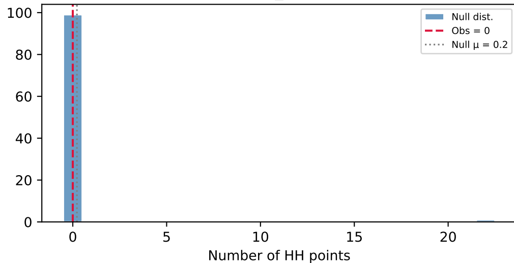
HH count (p_emp=1.000)
