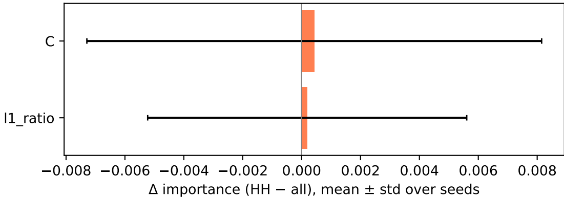
adult — LogReg
