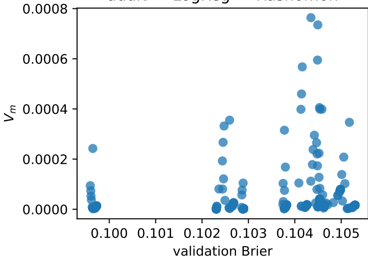
adult — LogReg — Rashomon
