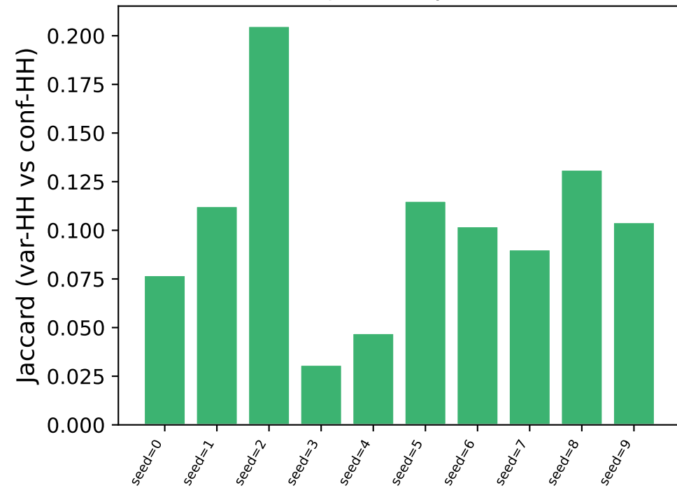
Cross Jaccard per seed
