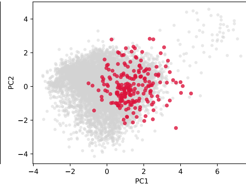
k=30, n_HH=217
