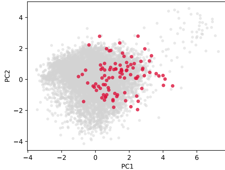
k=10, n_HH=93
