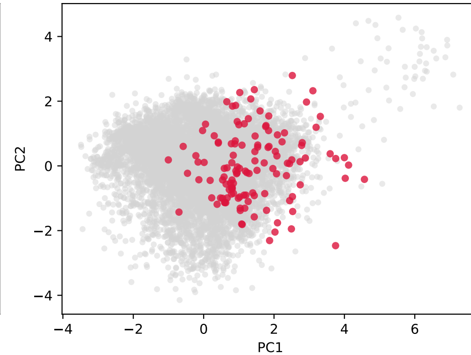
k=20, n_HH=124
