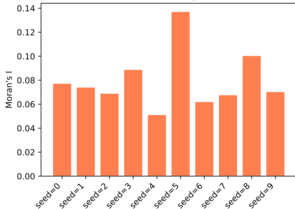
Global Moran's I per run
