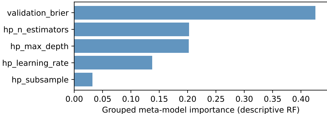
compas — GBM — Rashomon
