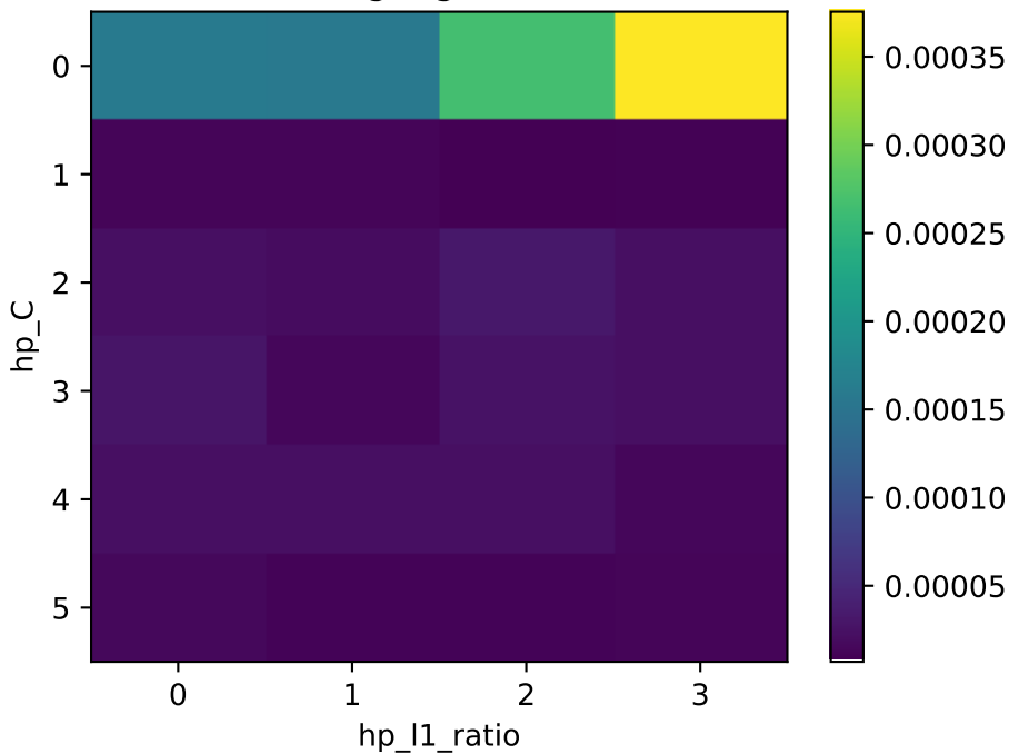
adult — LogReg — Rashomon
