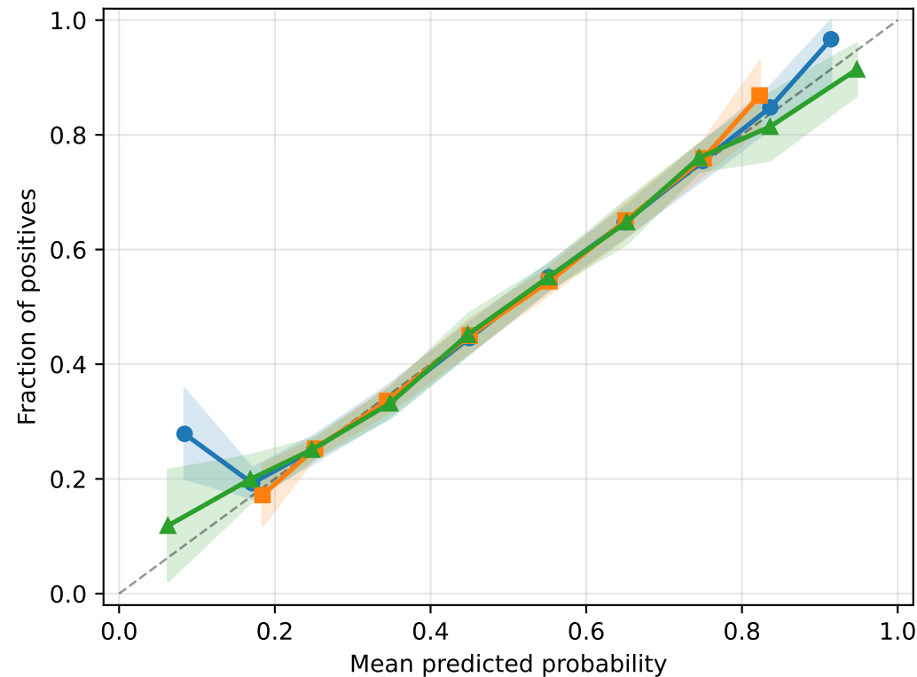
GBM (mean n=12.0)
