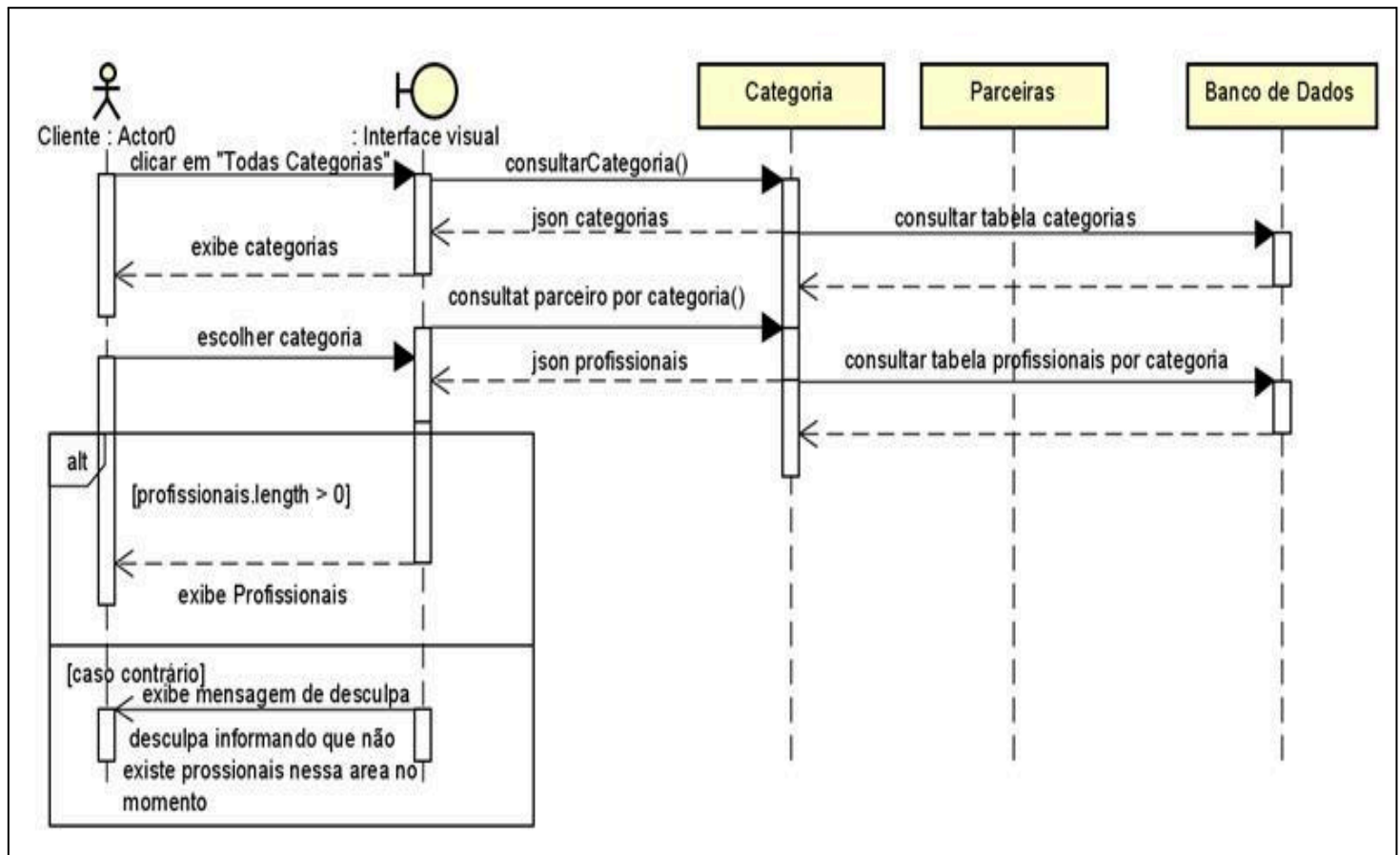
Figura 12 - Diagrama de Sequência I Fonte: Autoria Própria
