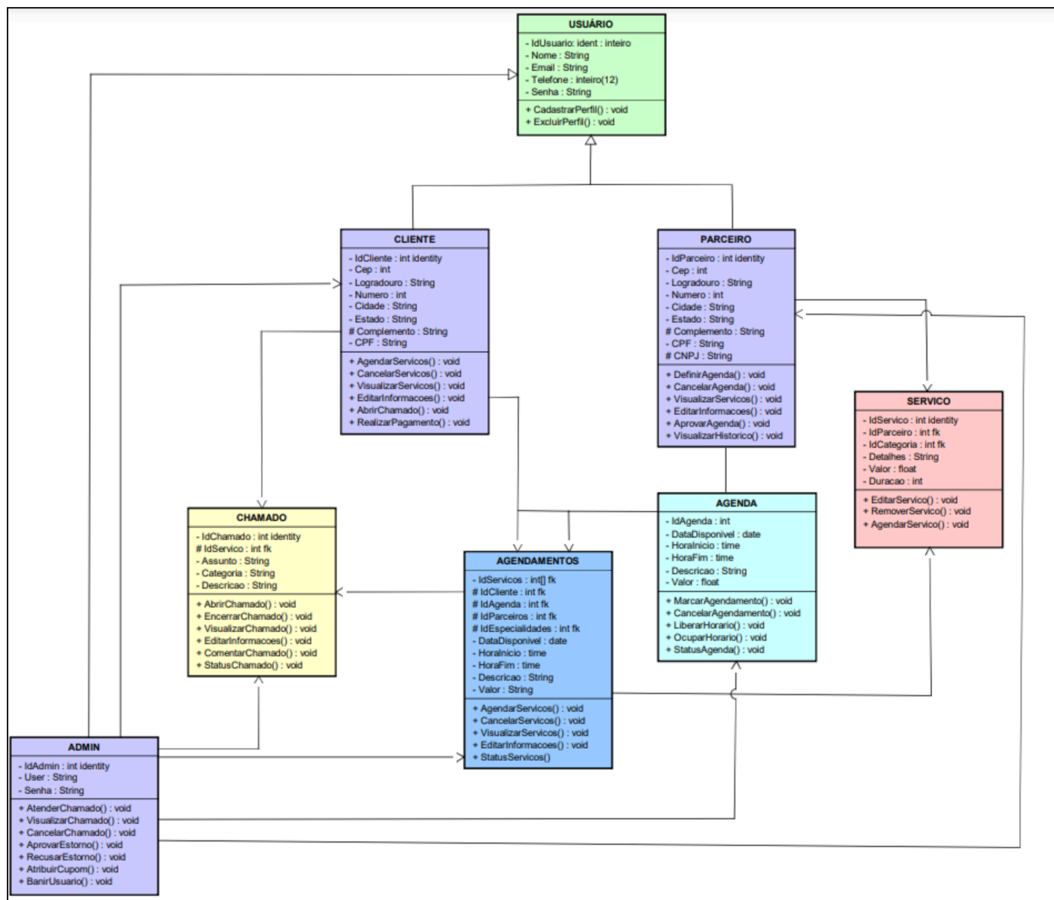
Figura 7 - Diagrama de Classe Fonte: Autoria Própria
