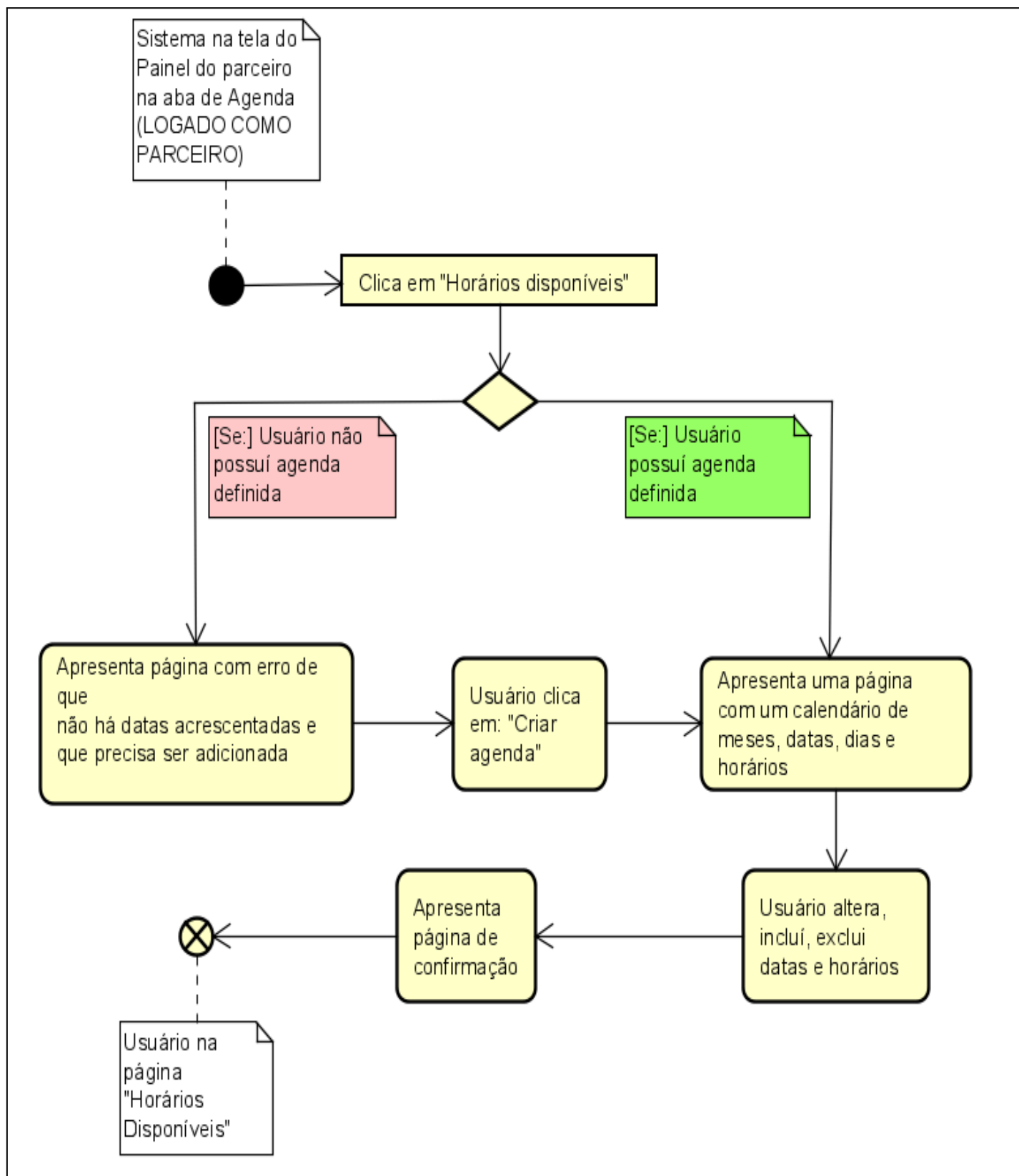
Figura 9 - Diagrama de Atividades II Fonte: Autoria Própria
