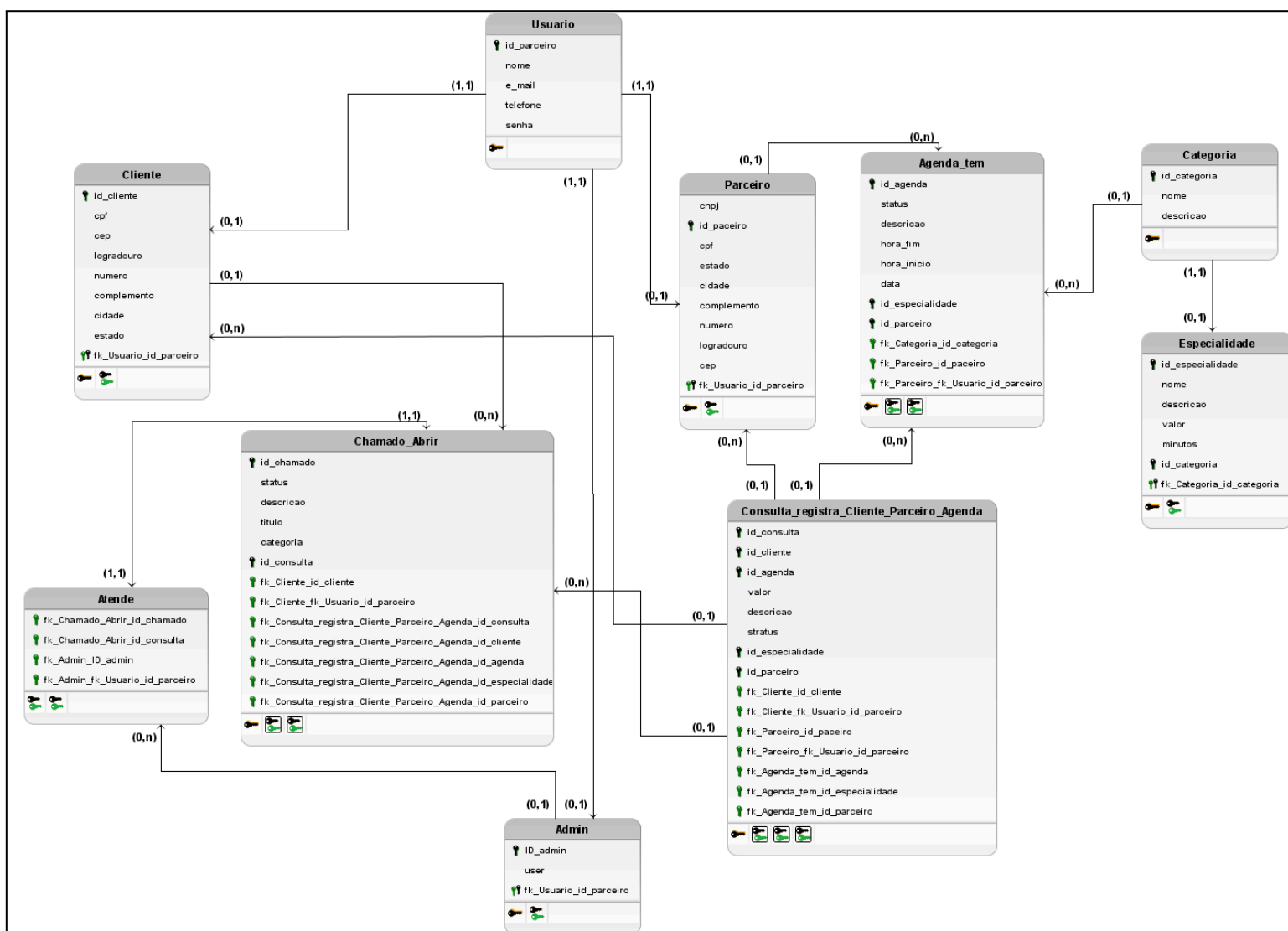
Figura 6 - Modelo Lógico Fonte: Autoria Própria
