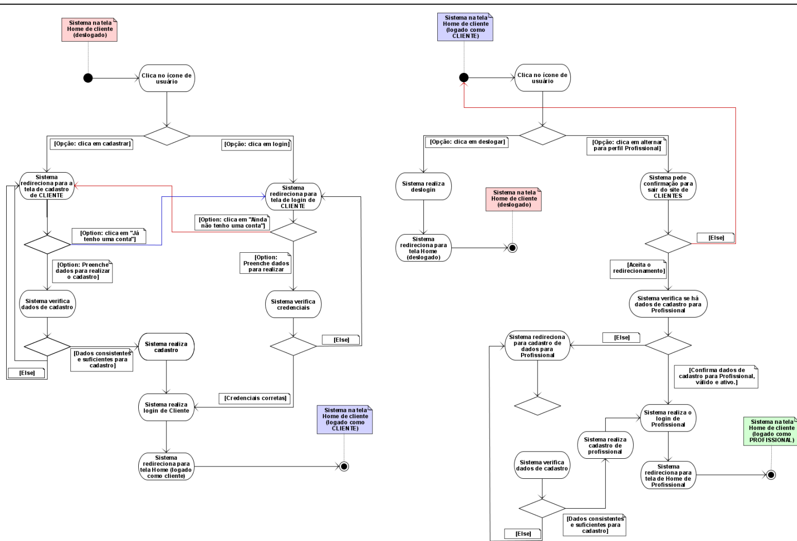
Figura 8 - Diagrama de Atividades I Fonte: Autoria Própria
