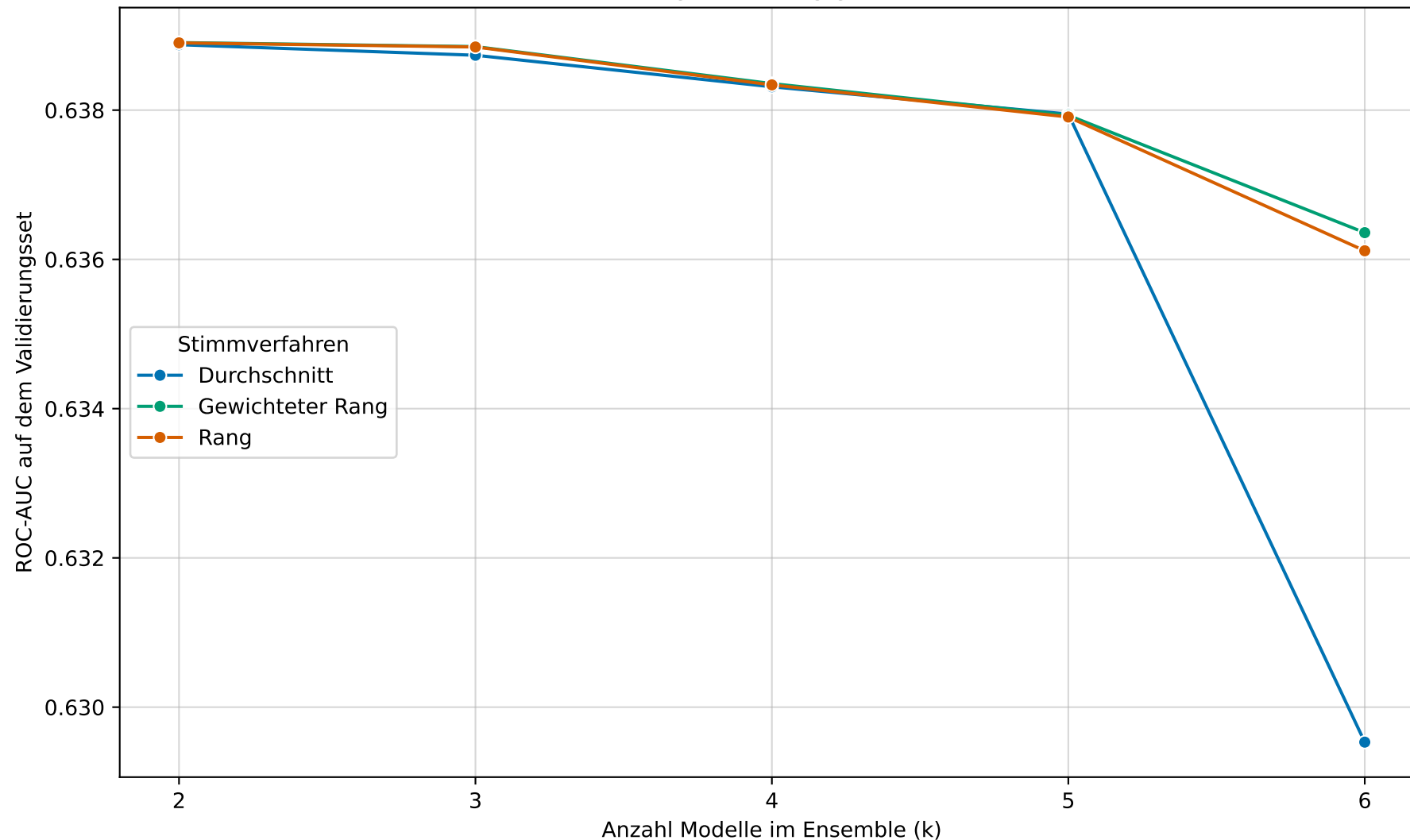
Beste Ensemble-Leistung in Abhängigkeit von der Modellanzahl
