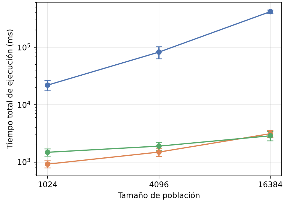
Mediana (1000 ítems)
