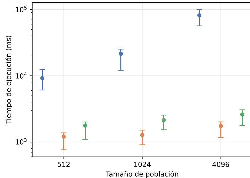
Mediana (1000 ítems)
