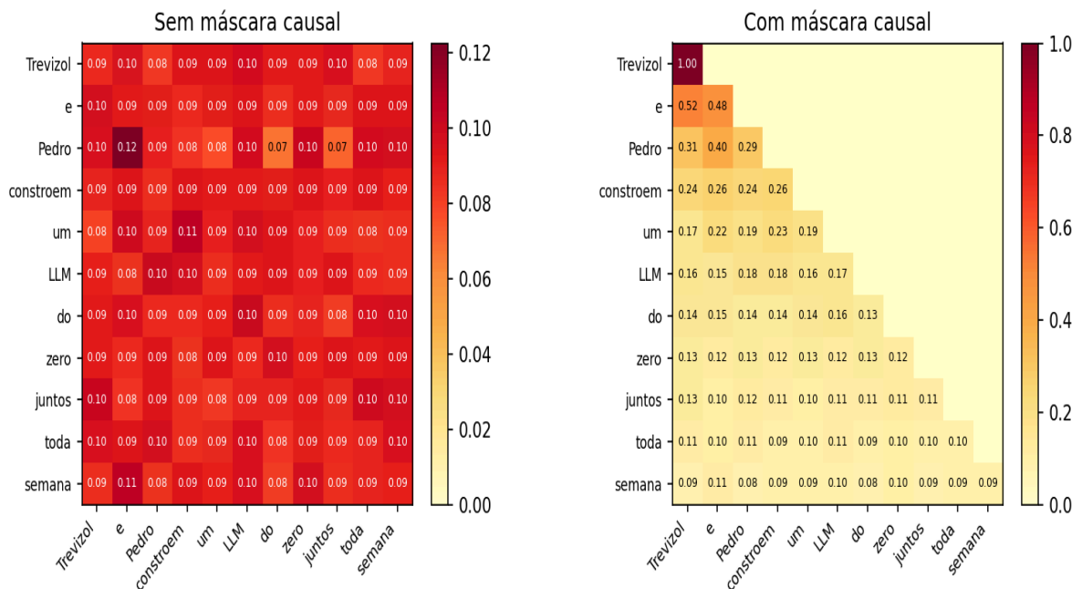
Matriz de atenção — "Trevizol e Pedro constroem um LLM do zero juntos toda semana"
