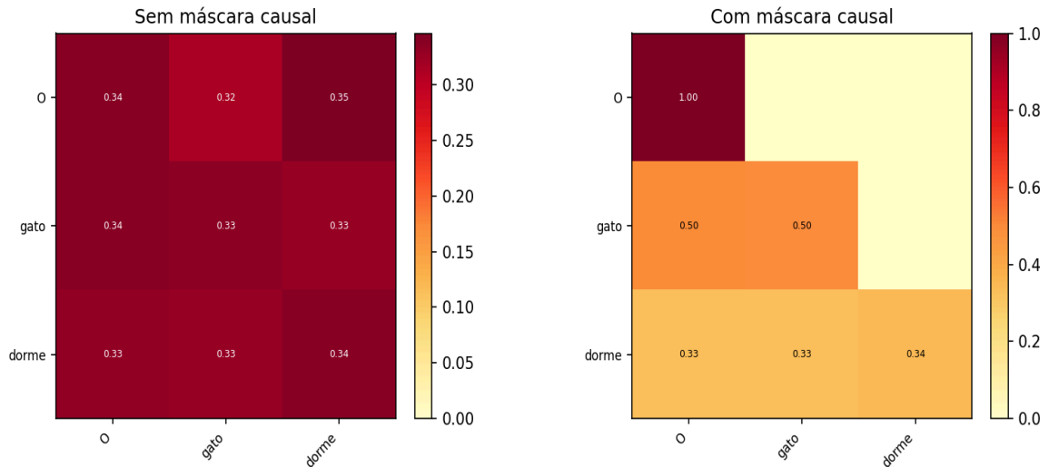
Matriz de atenção — "O gato dorme"
