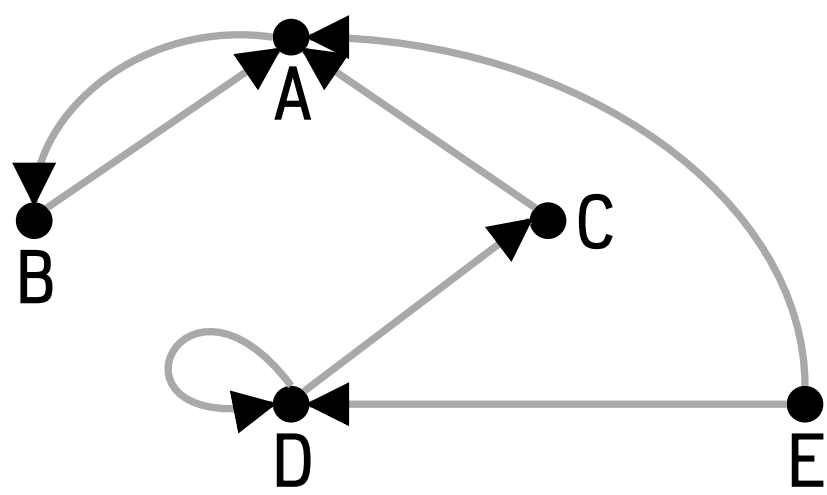
Gerichteter Graph - Beispiel
