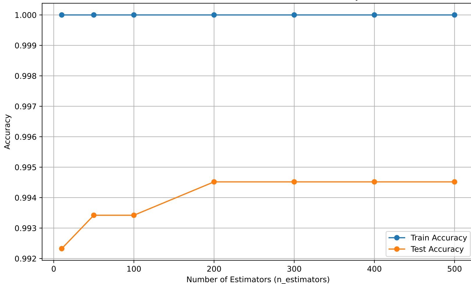
Influence du nombre d'arbres sur l'accuracy
