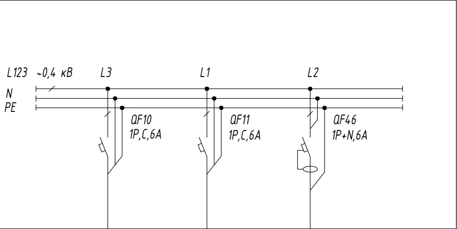
ВРУ (см. 25-05-3М)
