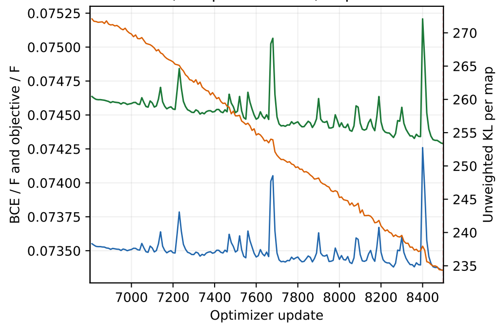
Stochastic train (10-update means) · updates 6801-8500
