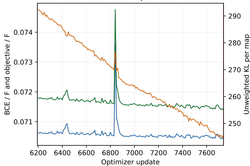
Posterior-mean train · updates 6193-7740
