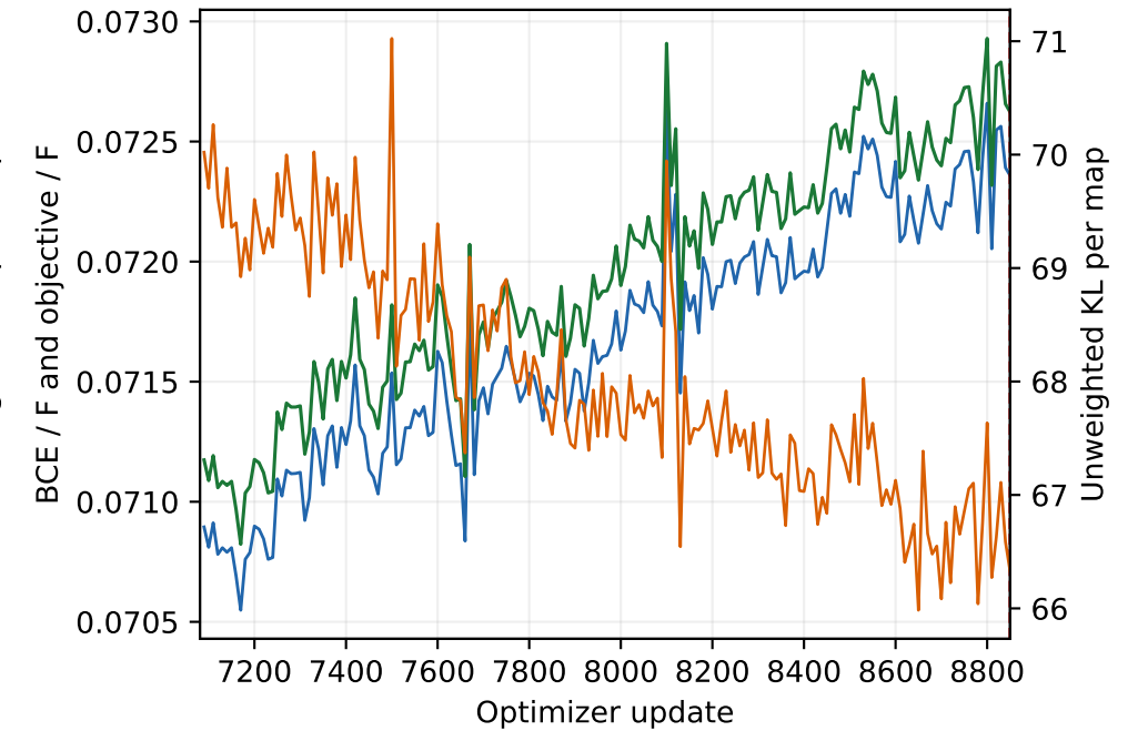
Posterior-mean validation · updates 7081-8850
