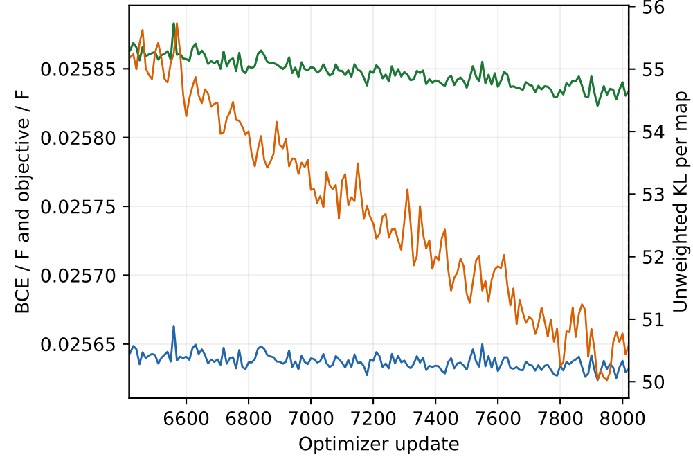
Posterior-mean train · updates 6417-8020
