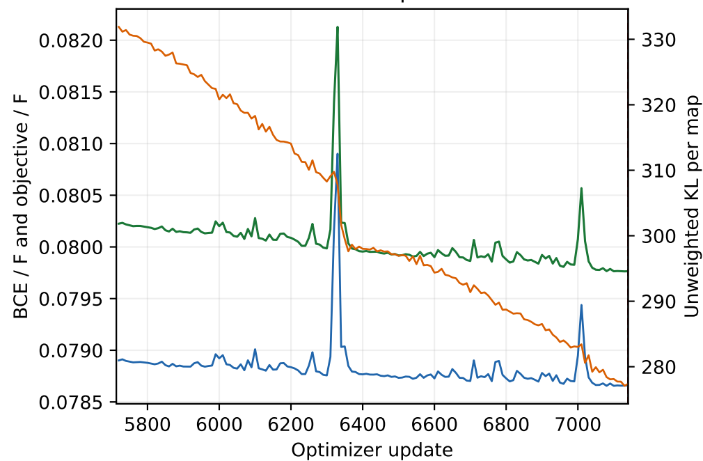
Posterior-mean train · updates 5713-7140
