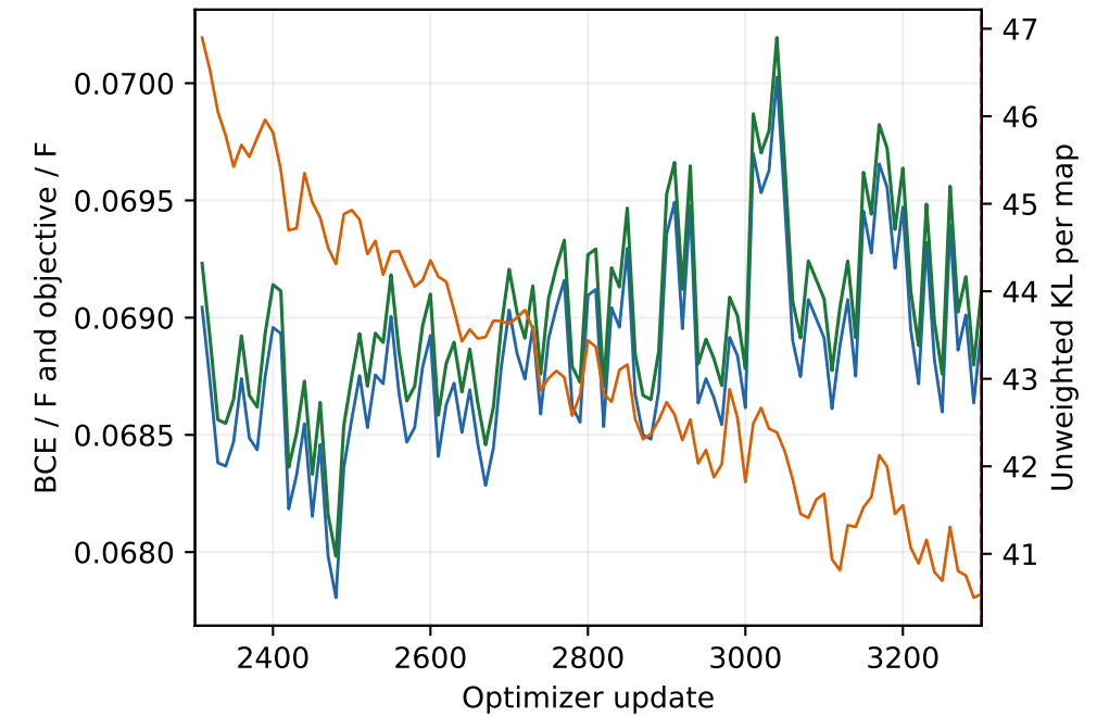
Posterior-mean validation · updates 2301-3300
