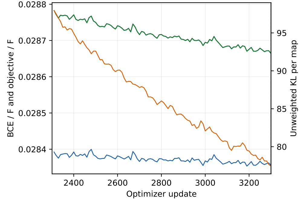
Posterior-mean train · updates 2301-3300
