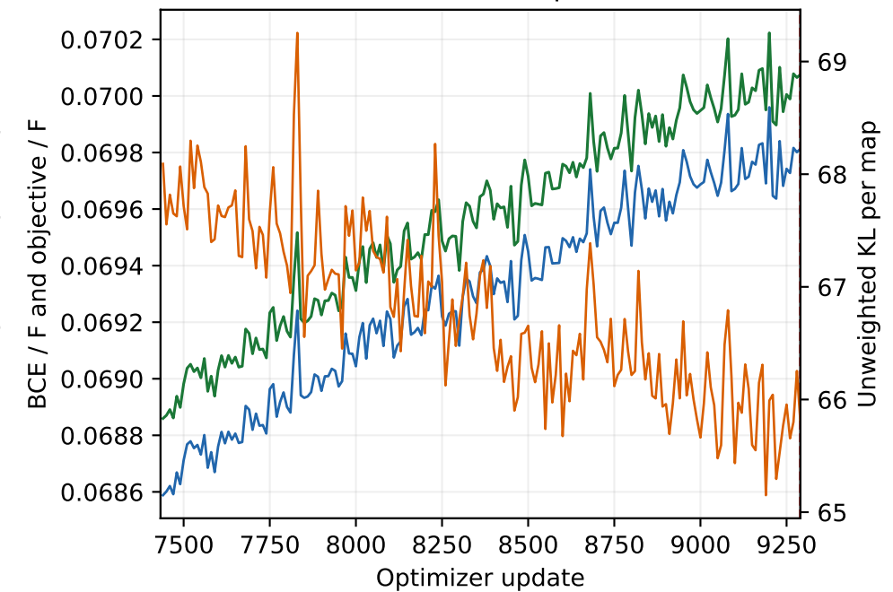
Posterior-mean validation · updates 7433-9290
