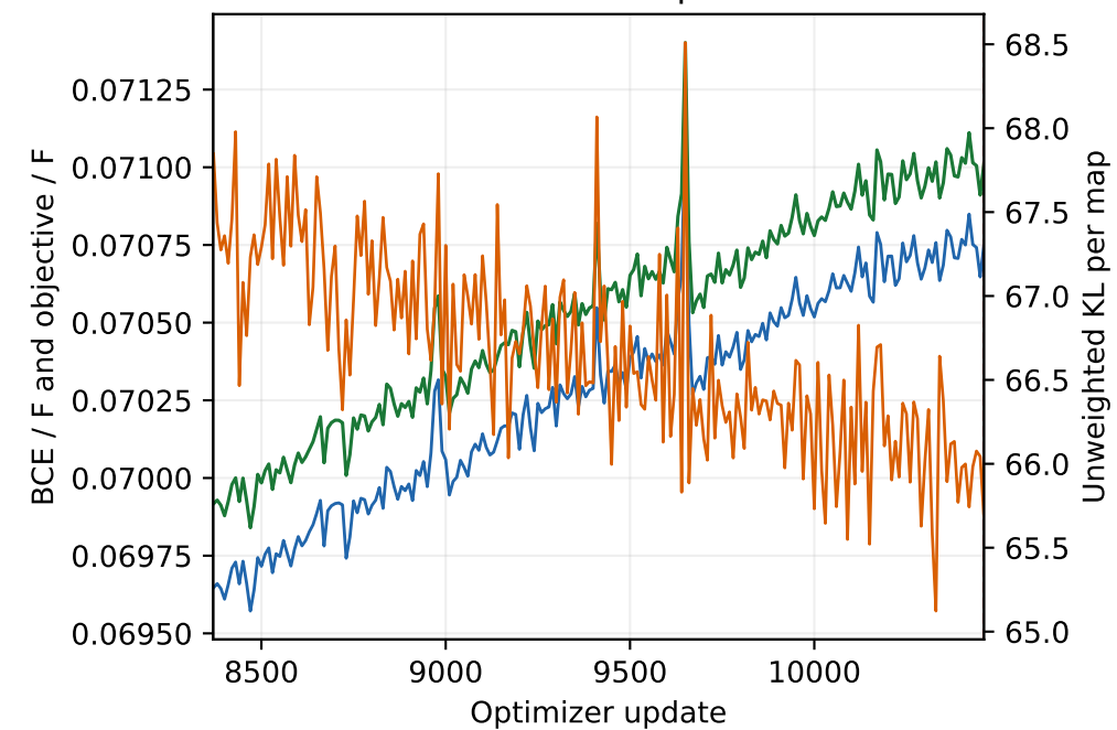
Posterior-mean validation · updates 8369-10460
