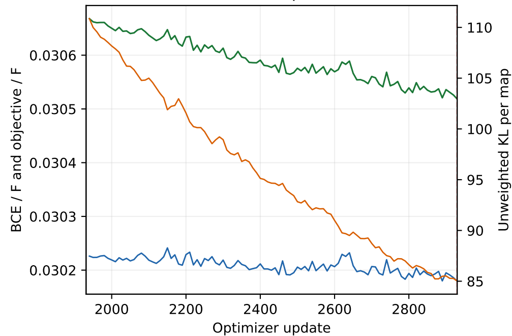
Posterior-mean train · updates 1931-2930
