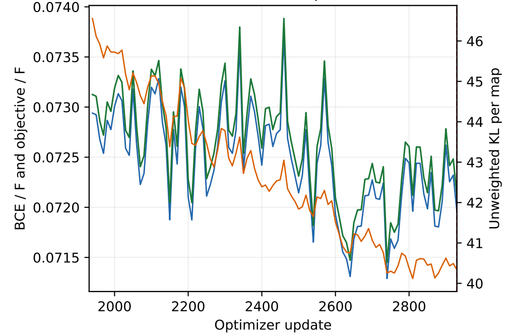
Posterior-mean validation · updates 1931-2930
