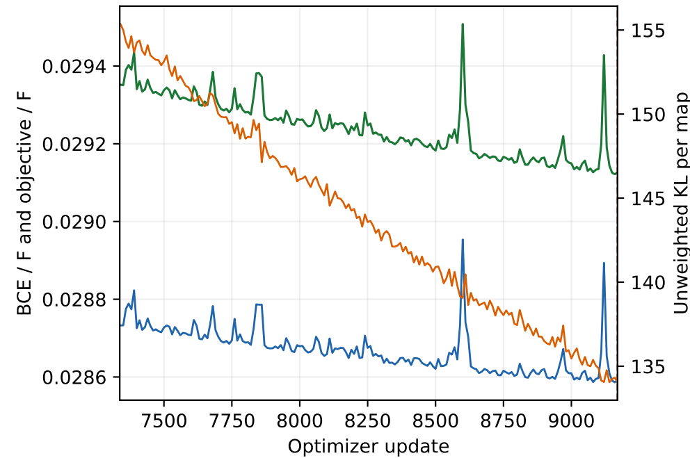
Posterior-mean train · updates 7337-9170
