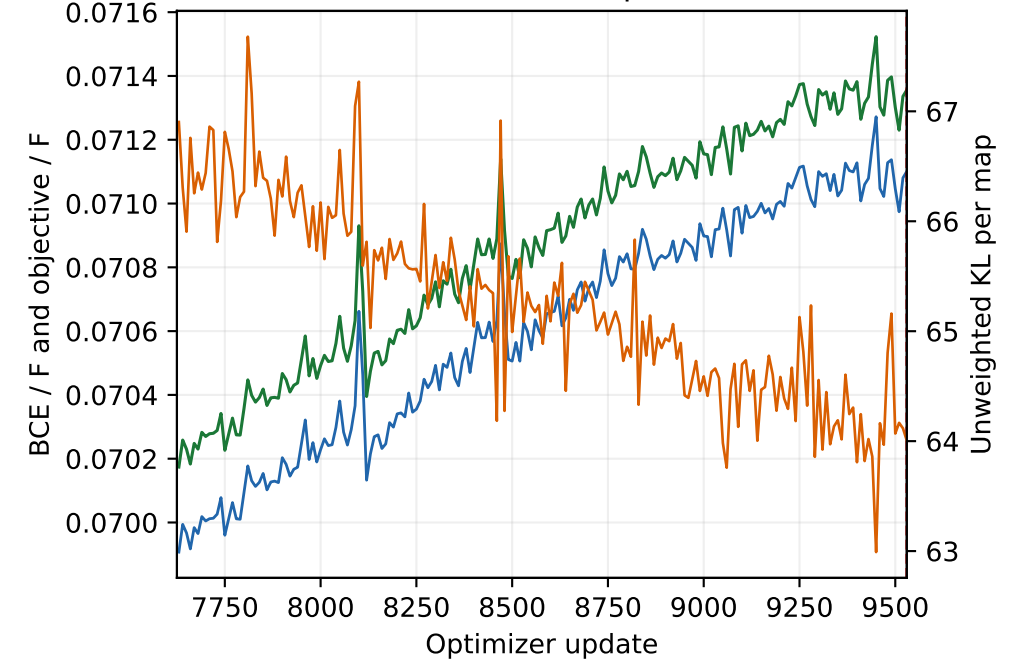
Posterior-mean validation · updates 7625-9530
