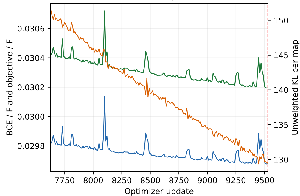
Posterior-mean train · updates 7625-9530
