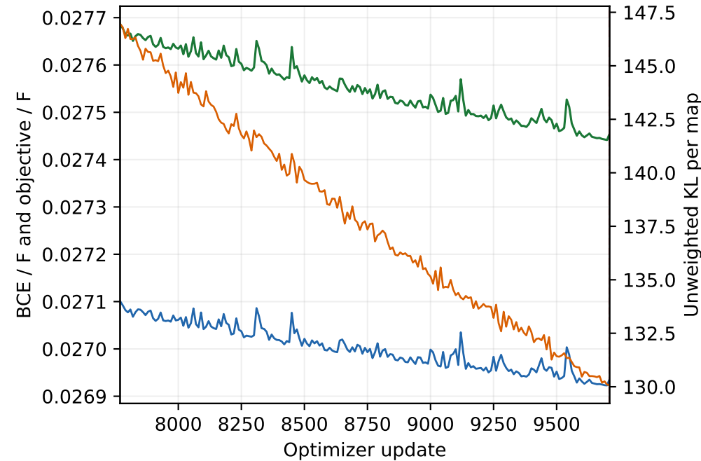
Posterior-mean train · updates 7769-9710
